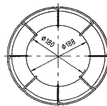
Bobina 76 Bobina metallica Foro dia. 180 mm Filo spira normale EN 759: K300
