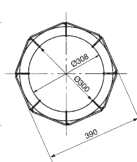
Bobina 28 Eurospool ® ottagonale Foro dia. 300 mm Filo spira-spira
