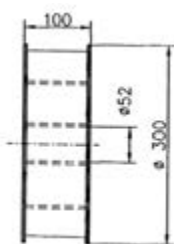
Bobina 66 ramata Cestello metallico Filo random
